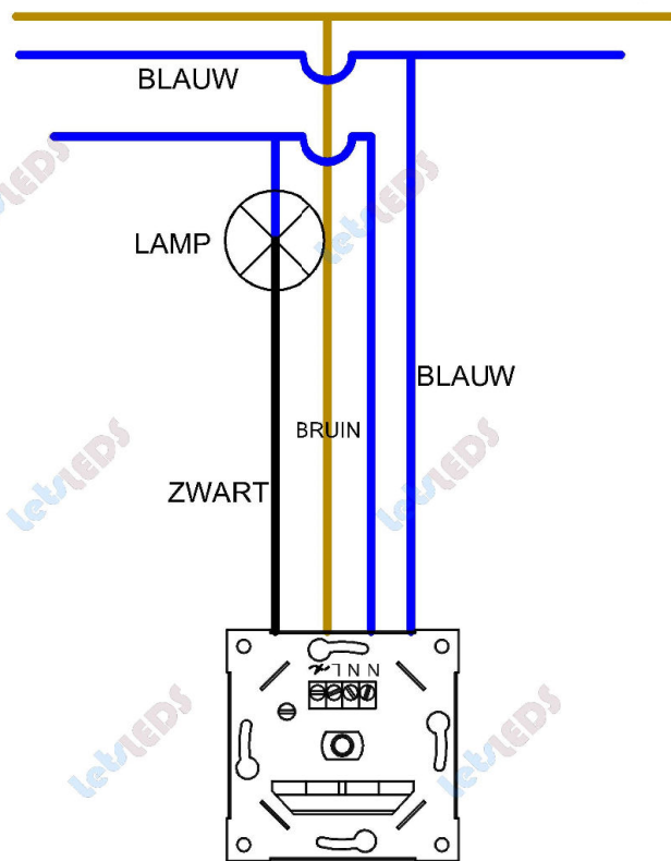
enkele schakeling
