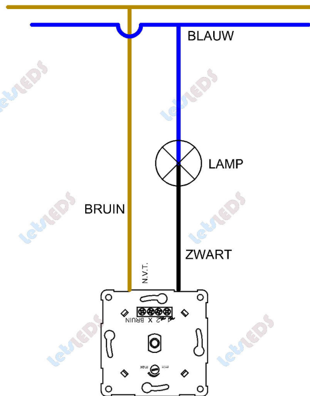
enkele schakeling
