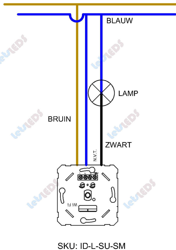
enkele schakeling
