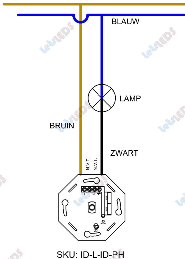
enkele schakeling
