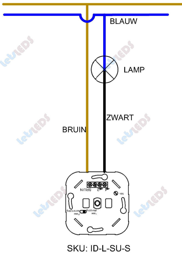
enkele schakeling
